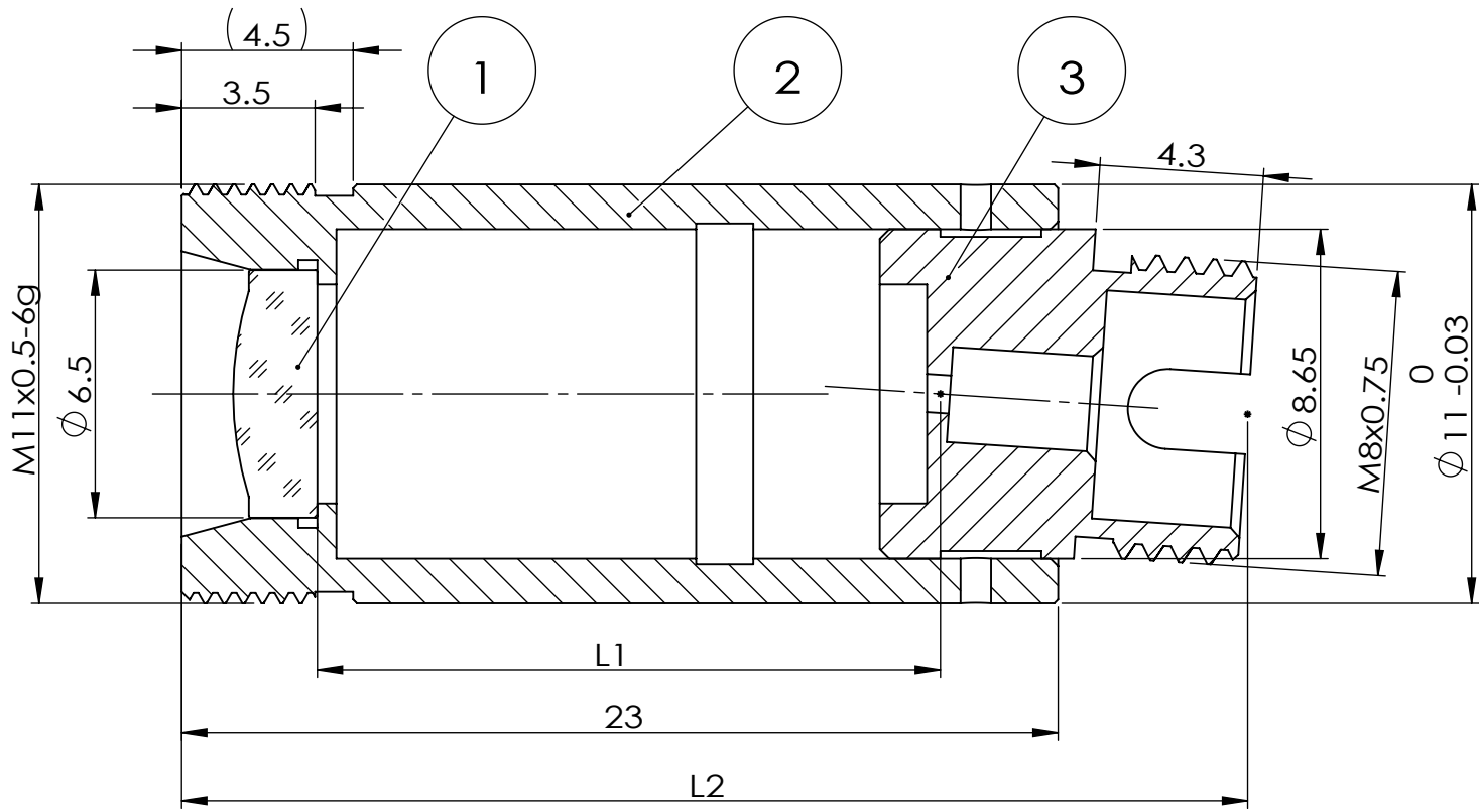
SECTION A-A
