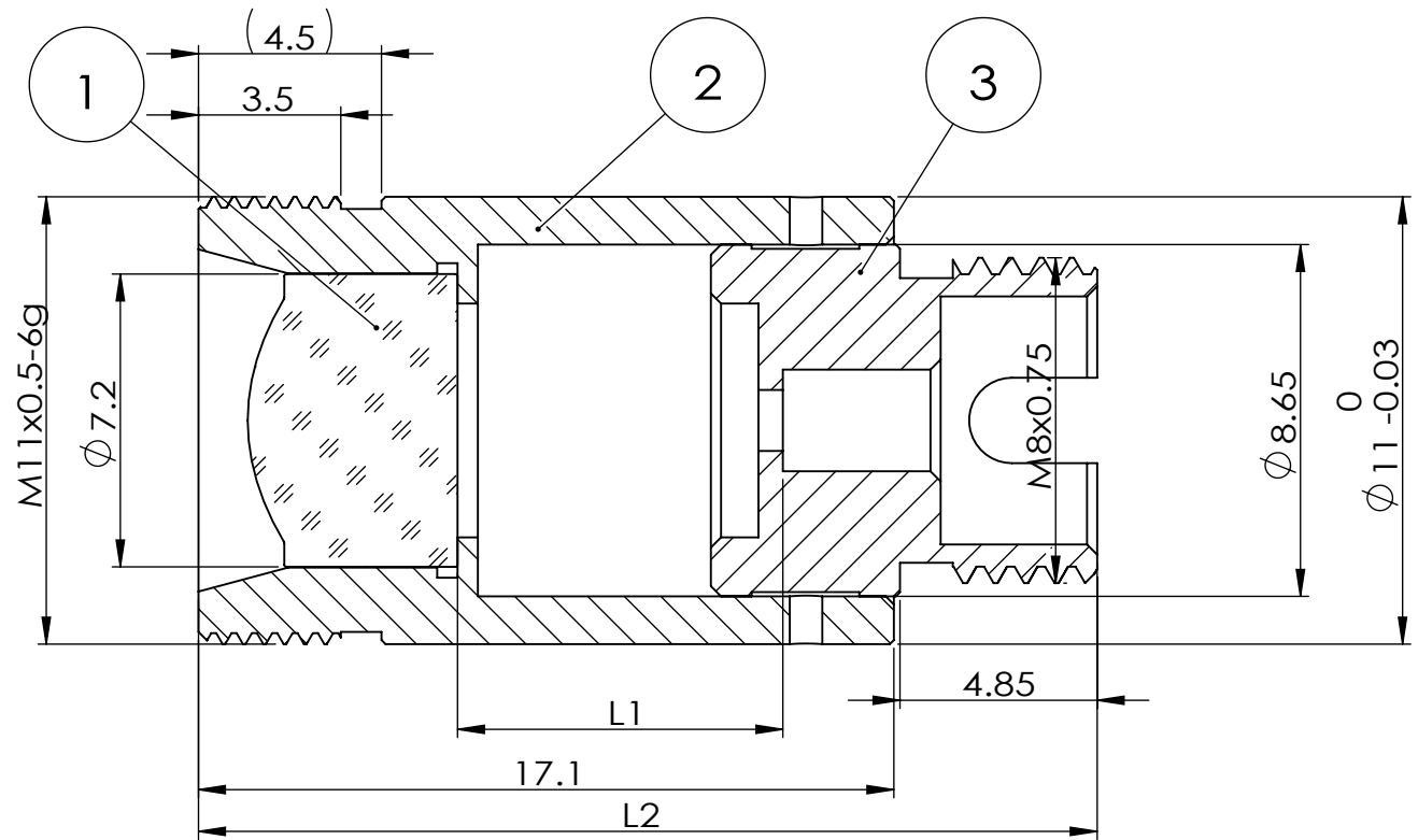
SECTION A-A
