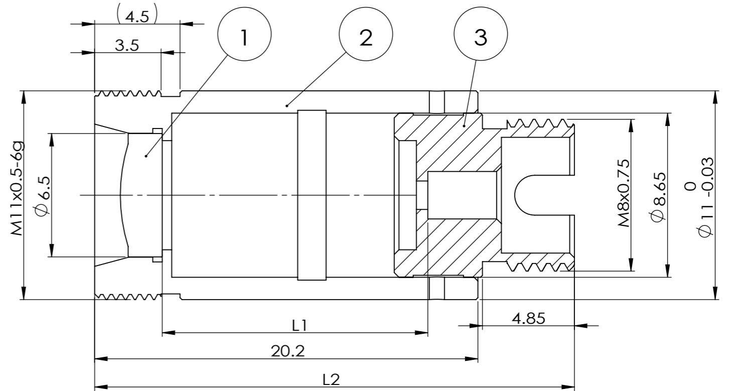
SECTION A-A
