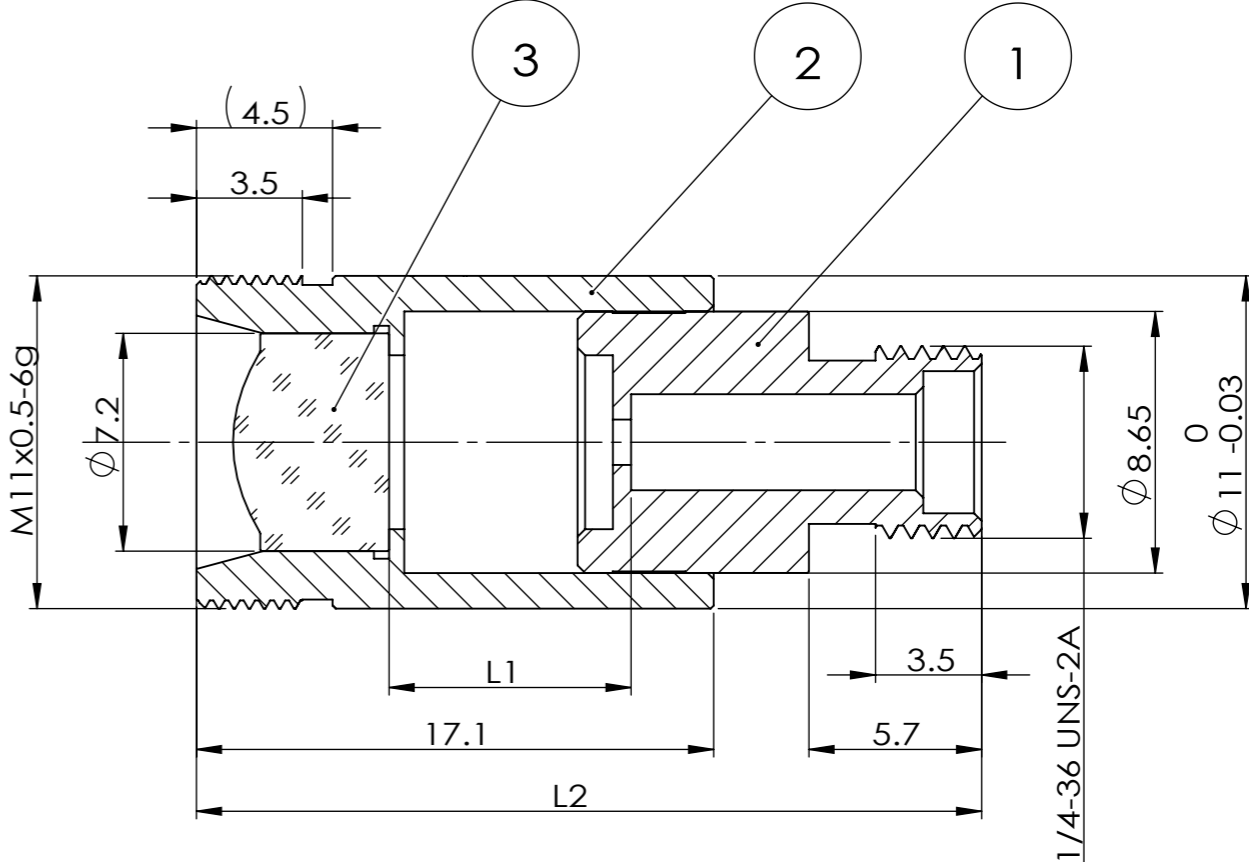
SECTION A-A
